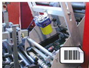
バーコードコントロールカメラ
